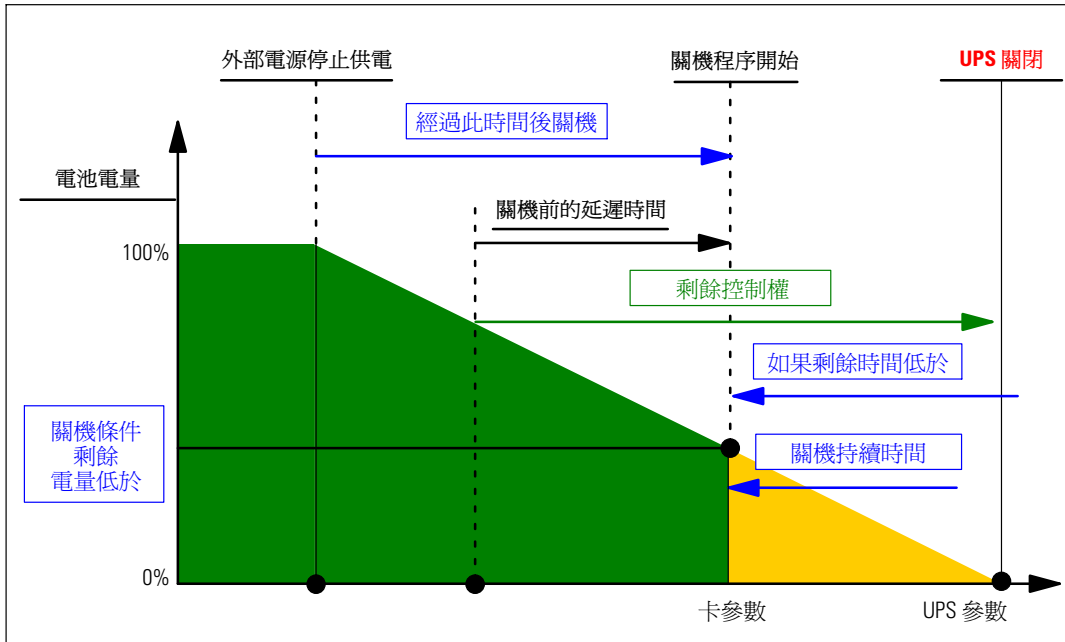
圖 48. 關機程序
